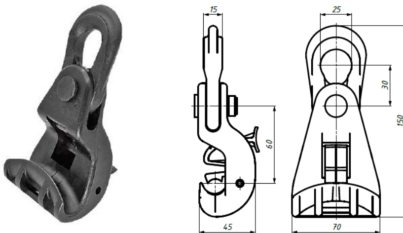
Рис. 1. Внешний вид поддерживающих зажимов PS 1500.
