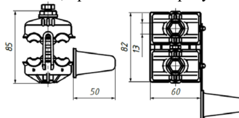
Рис. 1. Внешний вид герметичных ответвительных зажимов RP 150.
